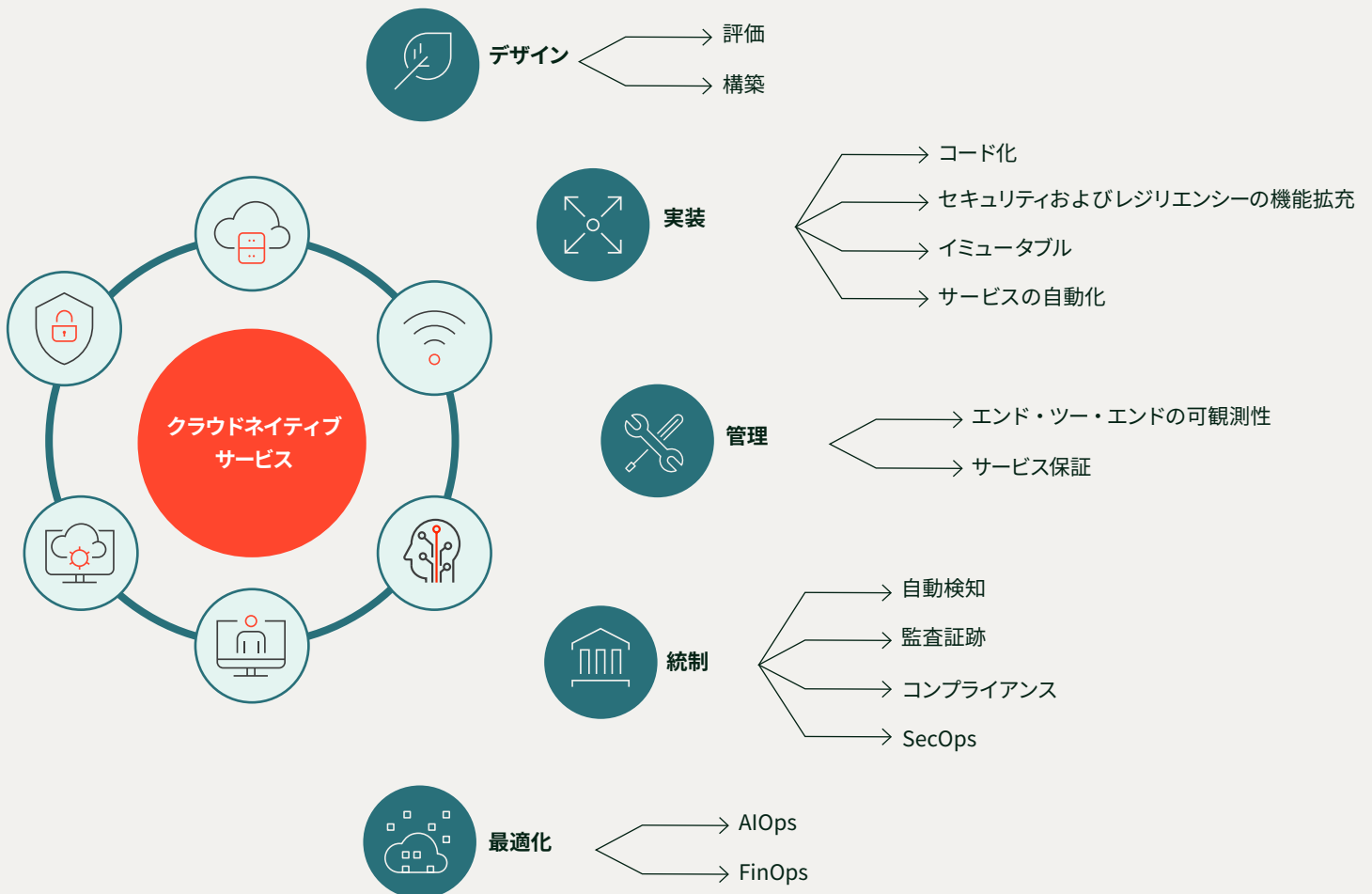
図 1. クラウドネイティブ運用フレームワークの実現
